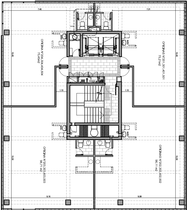
01 PLANTA PISOS 2, 3, 4 Y 5 Escala 1 : 75
