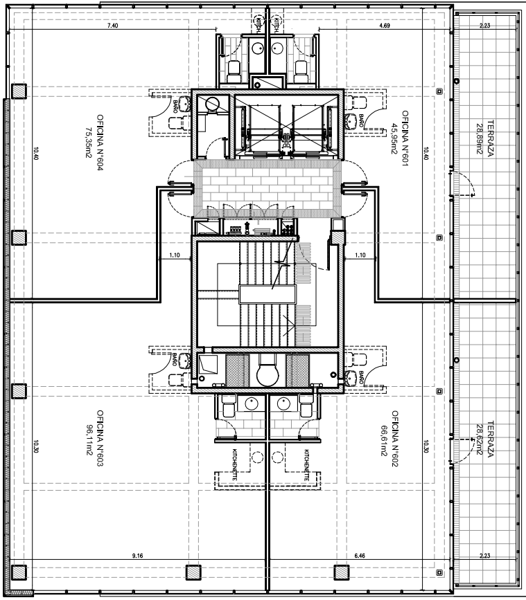
01 PLANIA PISO 6 Escala 1:75
